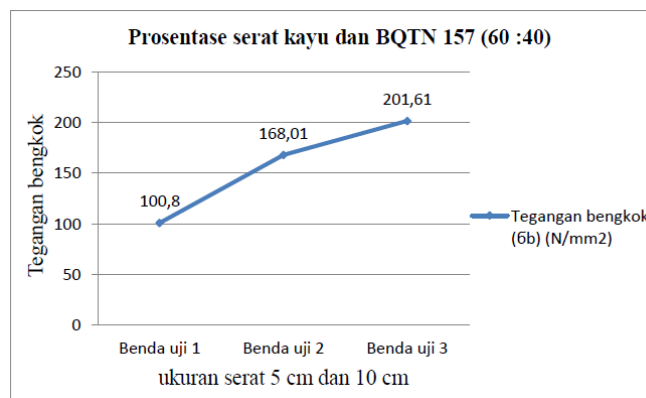
Gambar 2. Grafik Tegangan Bengkok Prosentase 20 : 80
