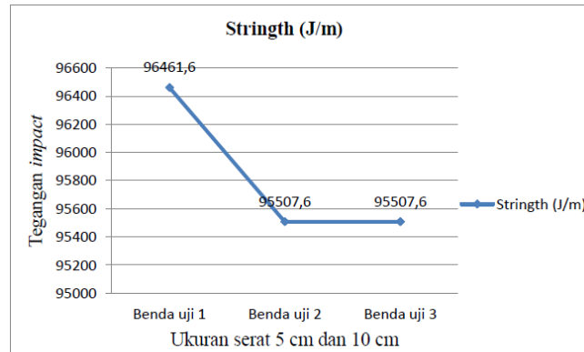
Gambar 1. Grafik Tegangan Impact Prosentase 20 : 80
